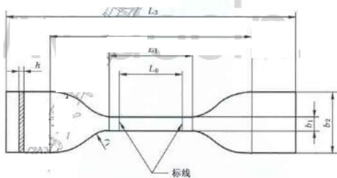
图 1 2 型试样
